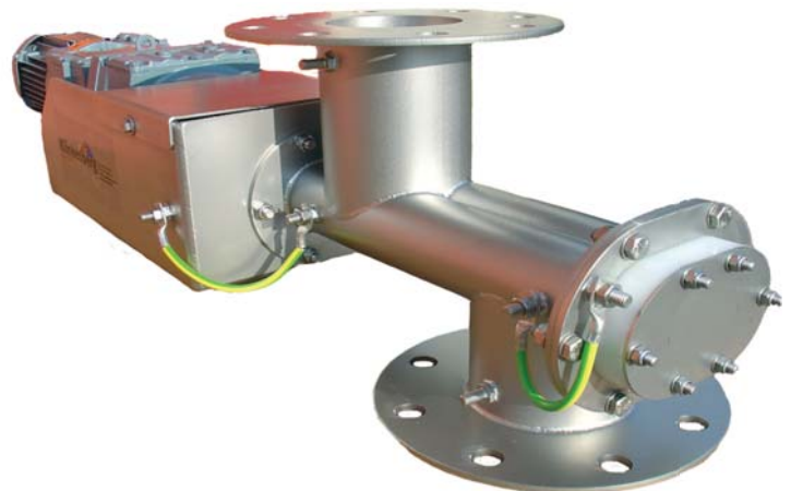
Doseerschroef voorzien van twee schroefassen zelfreinigend opgesteld.
